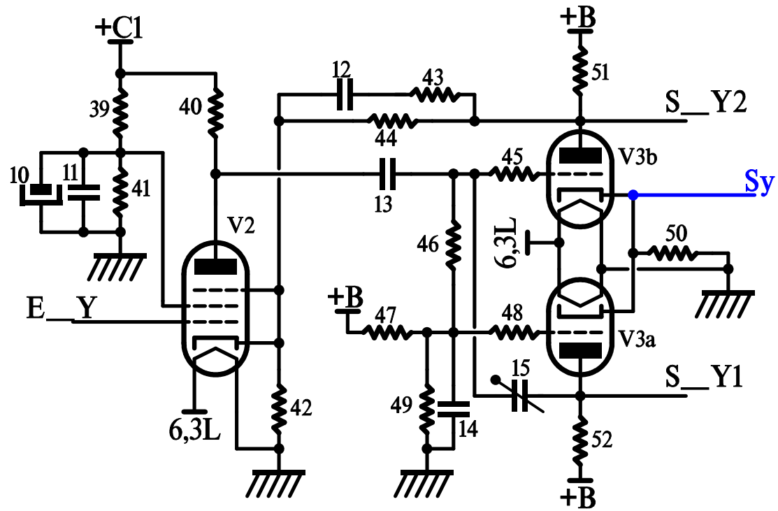
Amplificateur Vertical
