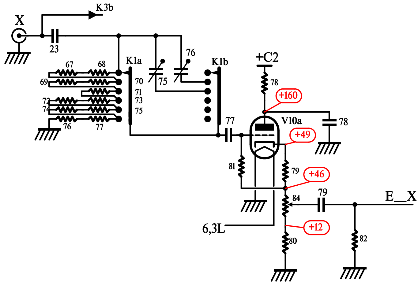
Atténuateur d'entrée horizontale
