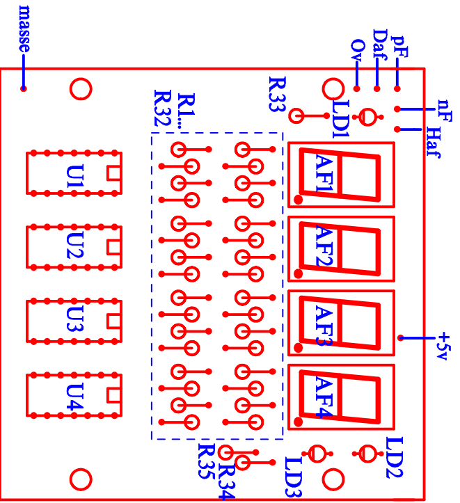
Carte afficheurs
