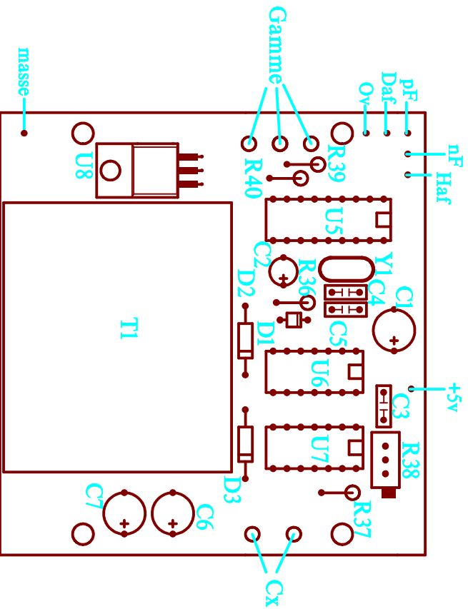
Carte alim-micro
