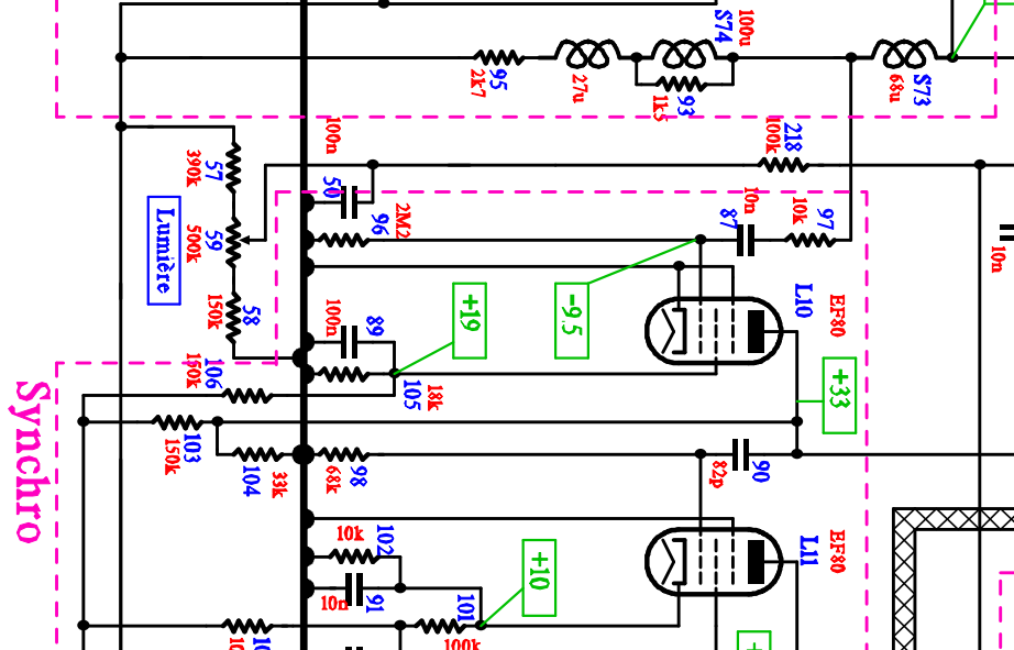
Amplificateur vidéo
